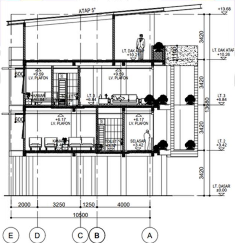
Potongan A-A
