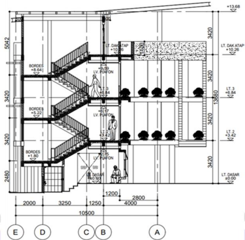
Potongan A-A
